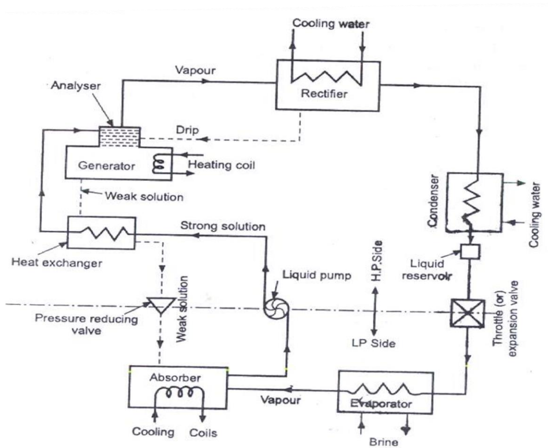
Fig. 4.1 Vapour Absorption System
